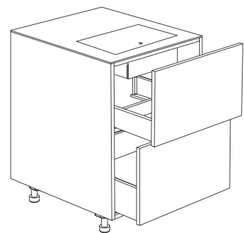
Módulo para fregadero. Sink base module 90 cm / 35" inch
